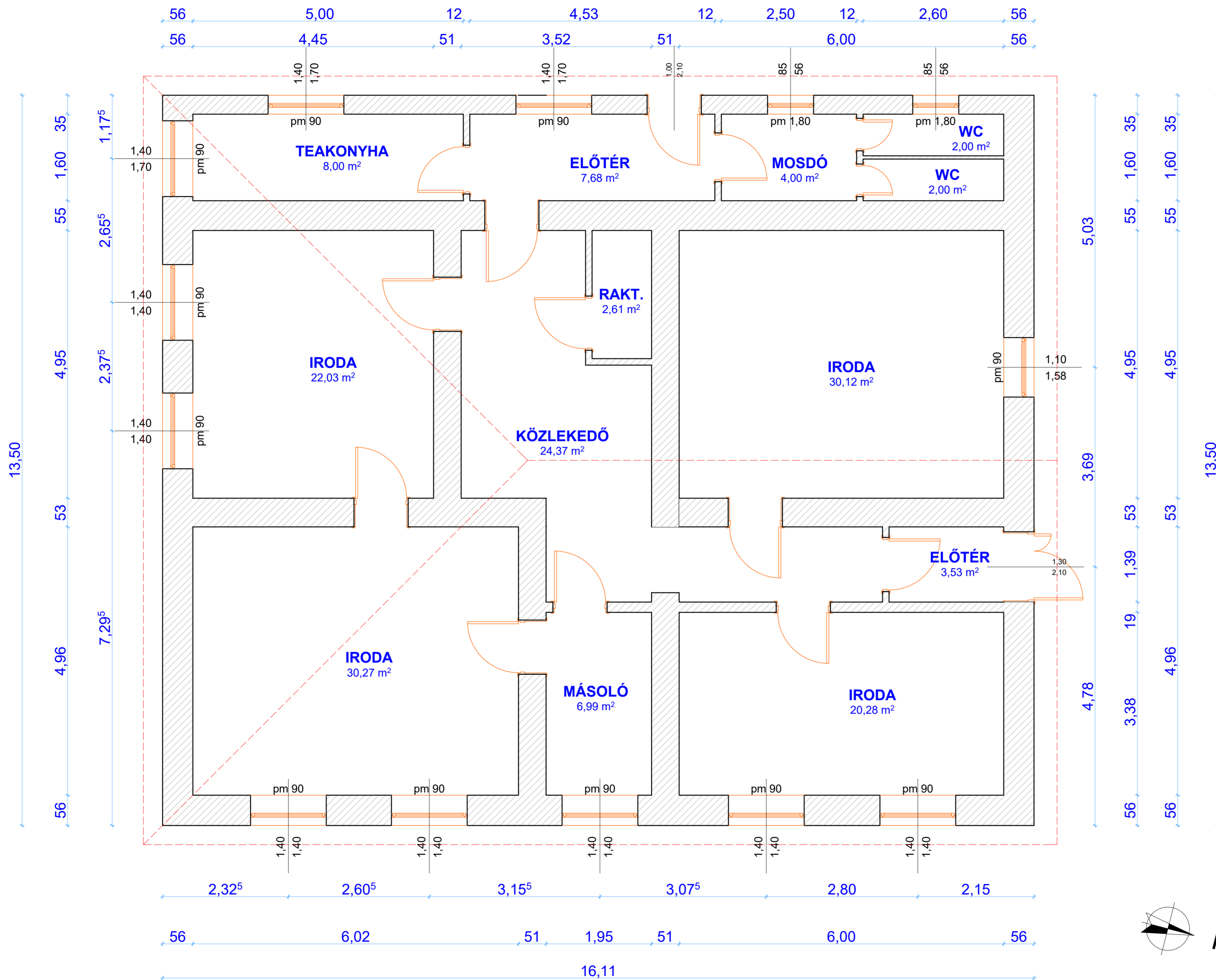
FELMÉRÉSI ALAPRAJZ M=1:50
